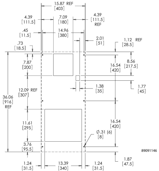
CUTOUT DIMENSIONS
